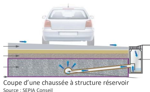
Coupe d'une chaussée à structure réservoir Source : SEPIA Conseil
