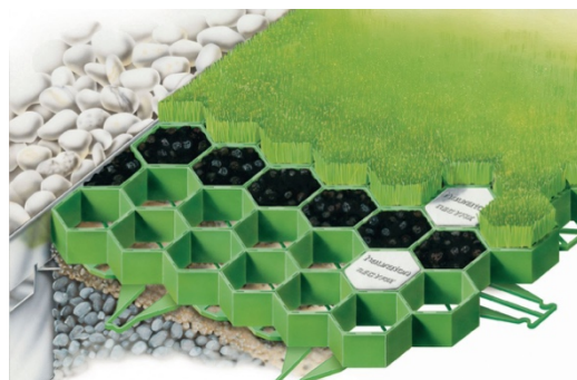
Module alvéolaire - Source : Hauraton France
