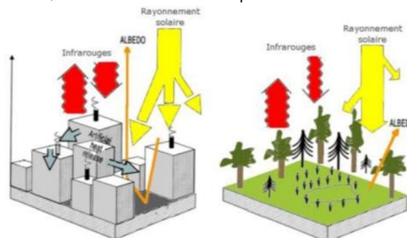
Flux d'énergie zone urbaine/zone rurale Source: Colombert, 2008
