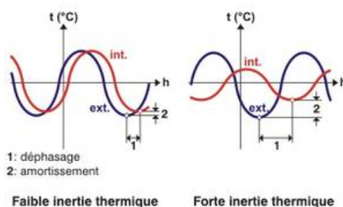
Inertie thermique d'un matériau Source : Manuel de bonnes pratiques architecturales - éco-construction et efficacité énergétique dans les bâtiments
