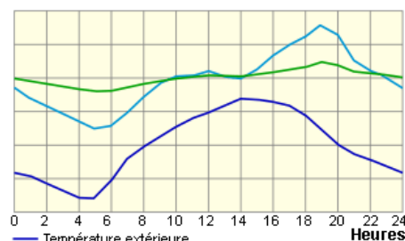
Bâtiment à forte et à faible inertie
