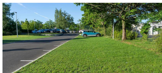
Parking végétalisé. Source : Ecovegetal
